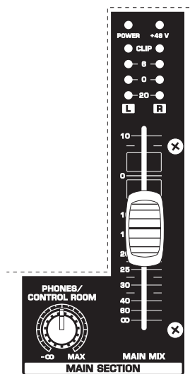
Рис. 2.10: Мониторный регулятор и фейдер Main Mix
