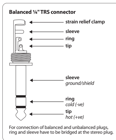
Рис. 3.3: 6,3-мм-стереохраповый штекер
