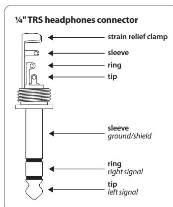
Рис. 3.4: Стереохраповый штекер для наушников
