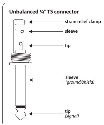
Рис. 3.2: 6,3-мм-монохраповый штекер
