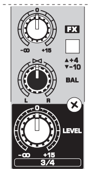
Рис. 2.6: FX Send/Balance/Level-регулятор
