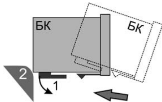
Рис. 3 Установка на “высокую” панель
