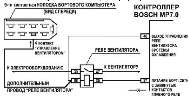
рис. 4 Аппаратное подключение функции “ТРОПИК”
